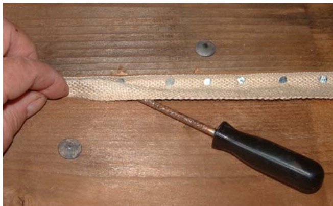
Foto B30 Het vorkje in gebruik om een "moet" in het band te zetten.
