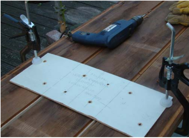
Foto B15 Mal omgeklapt, weer vastgeklemd en de gaten voor de middenklamp geboord.
